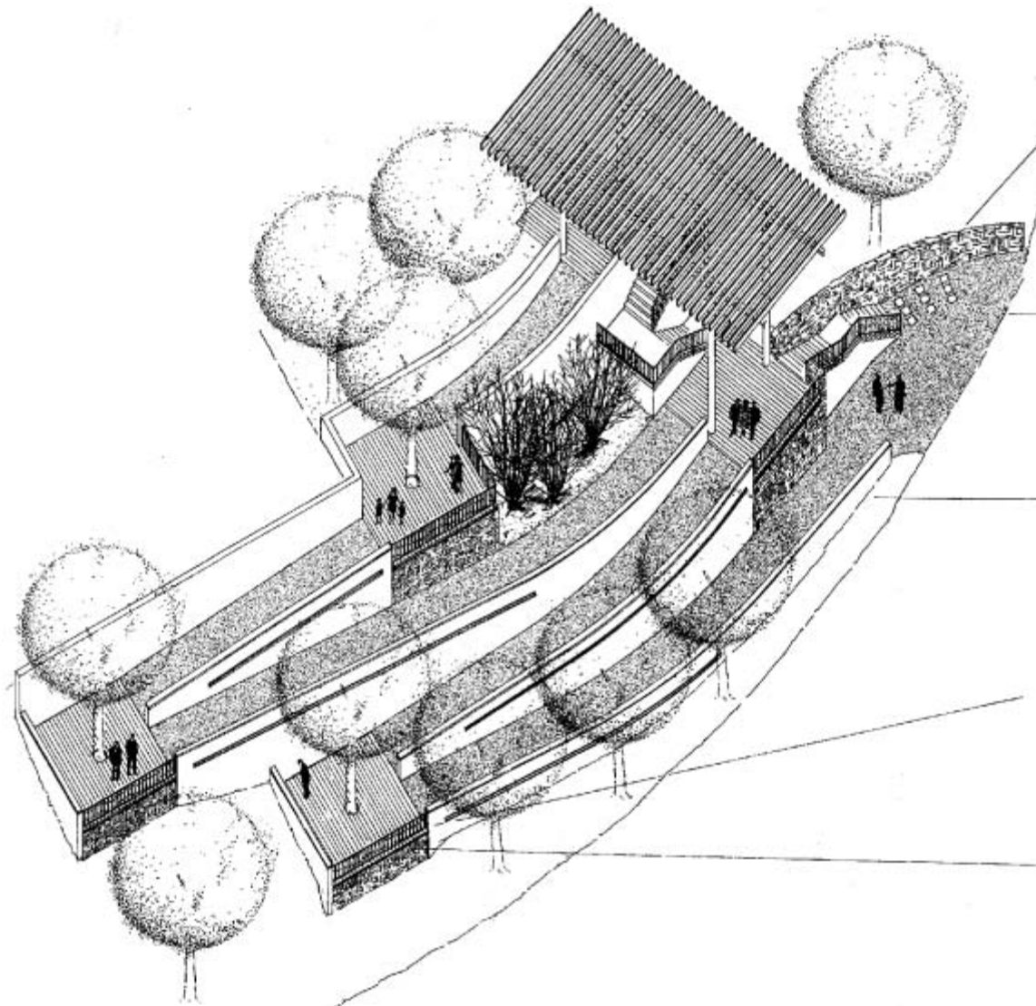
Stützmauern
